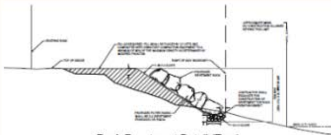
Rock Revetment Detail (Typ.) Scale: N.T.S.
